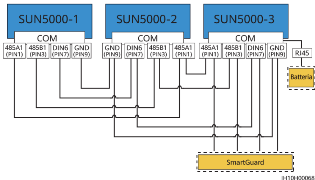
Figura 5-17 Collegamento in rete di SmartGuard (i riquadri tratteggiati indicano i componenti opzionali)
