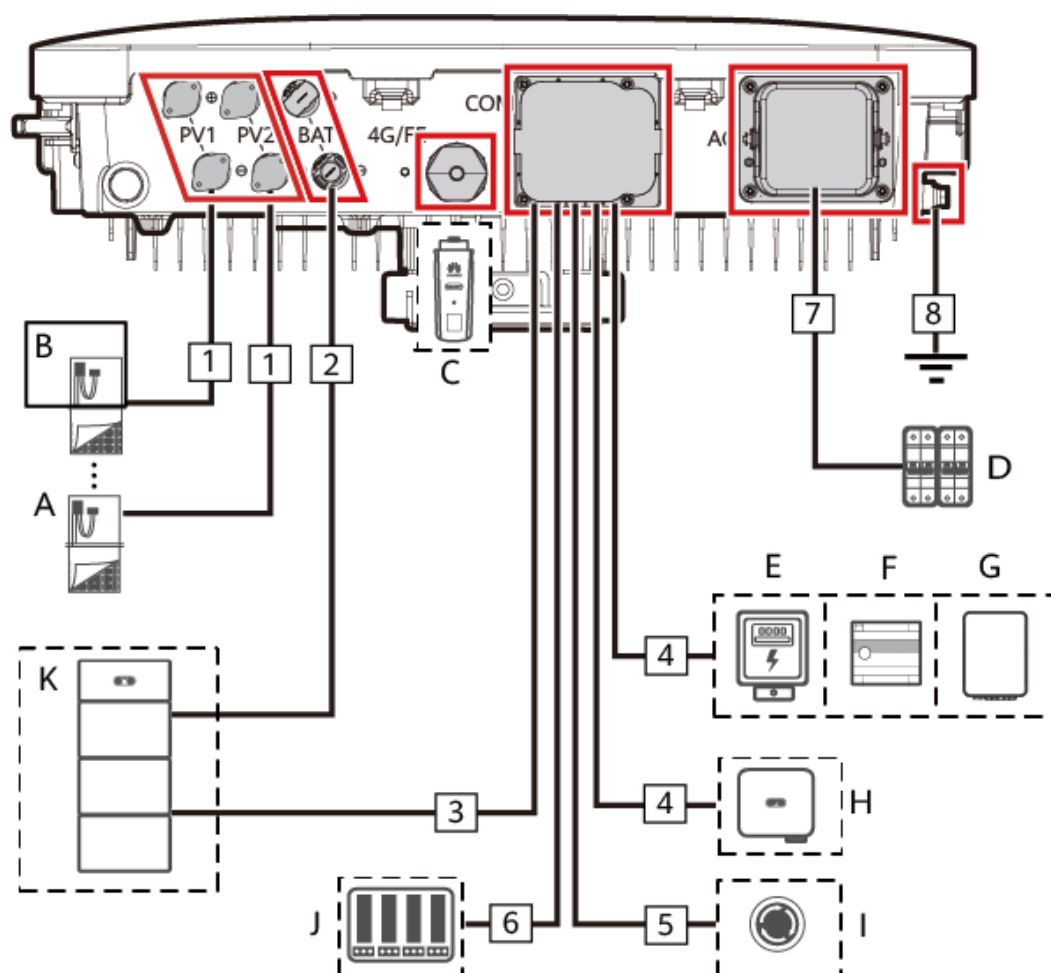
Figura 5-1 Collegamenti dei cavi del inverter (i riquadri tratteggiati indicano i componenti opzionali)
