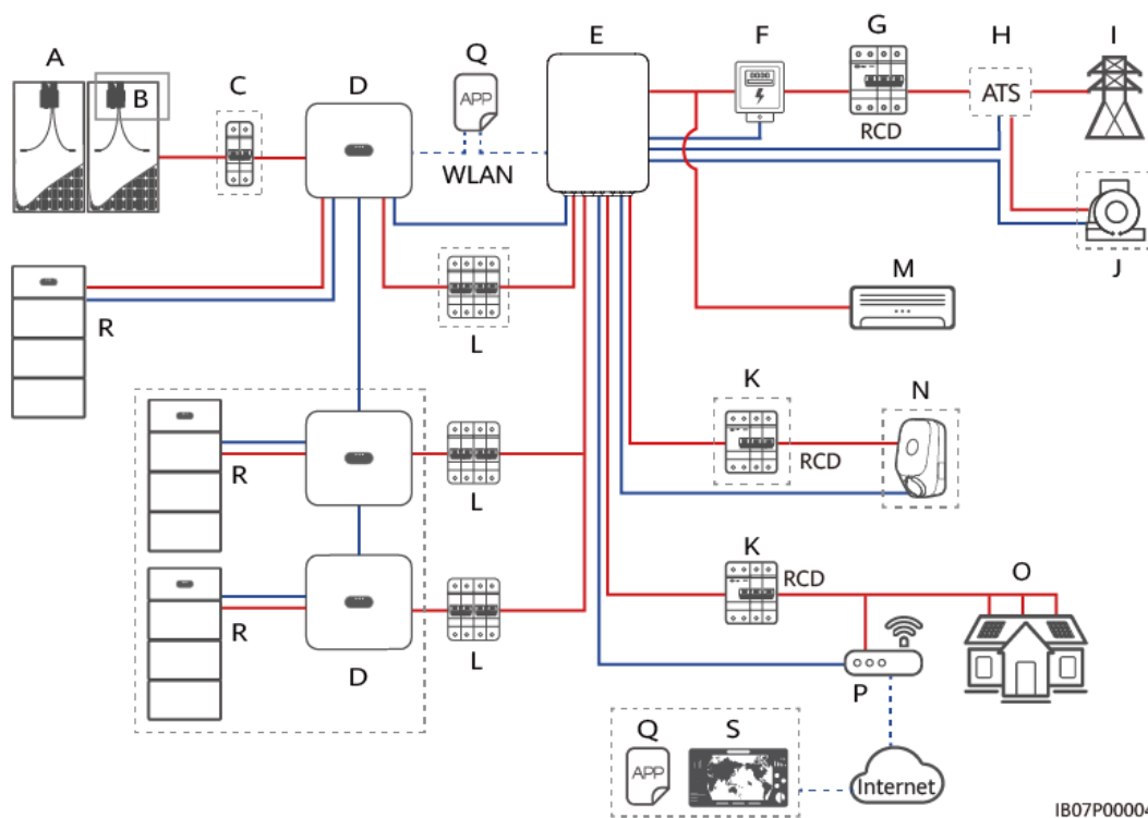
Figura 2-6 Collegamento in rete con alcuni dei carichi collegati a SmartGuard (i riquadri tratteggiati indicano i componenti opzionali)
