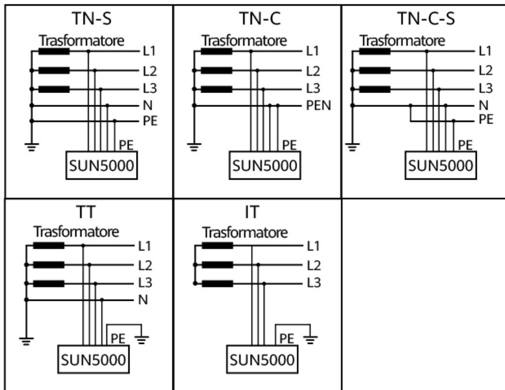
Figura 2-7 Sistemi di messa a terra
