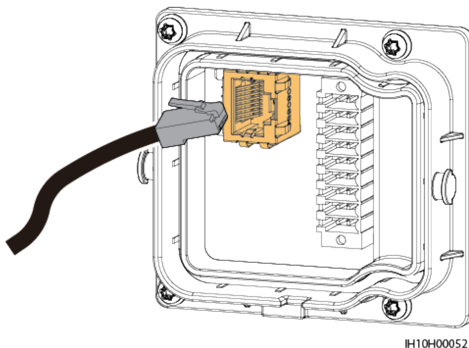
Figura 5-42 Installazione del cavo
