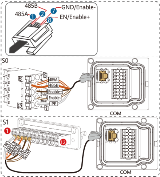
Figura 5-41 Collegamento cablato
