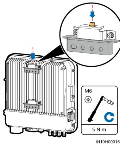
Figura 4-13 Installazione dell'inverter
