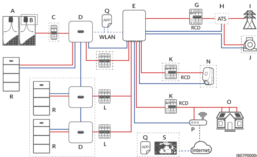
Figura 2-5 Collegamento in rete con tutti i carichi collegati a SmartGuard (i riquadri tratteggiati indicano i componenti opzionali)
