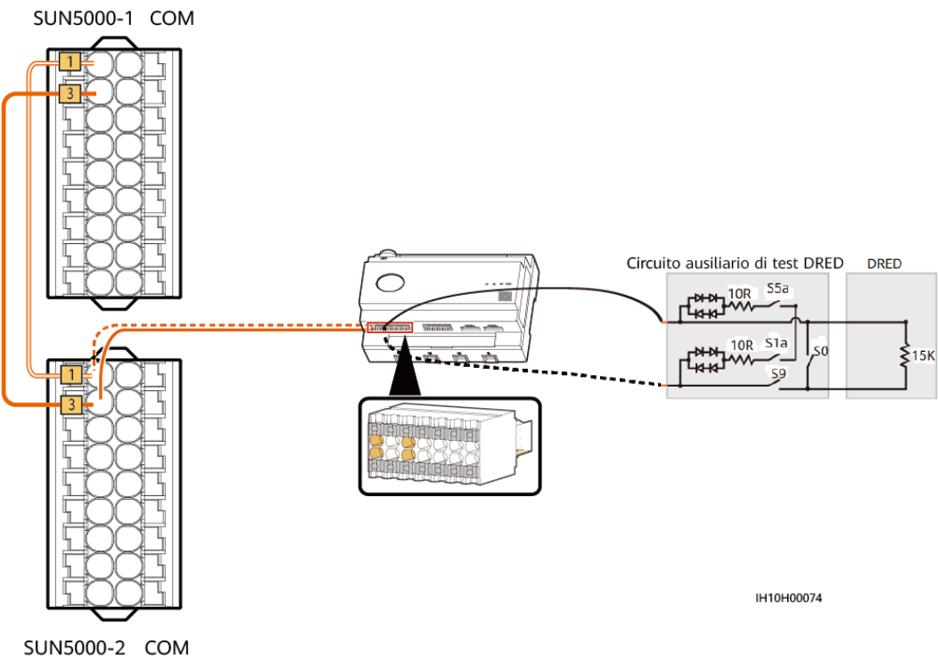
Figura 7-9 Schema di cablaggio per funzione DRM (collegamento in rete di EMMA)
