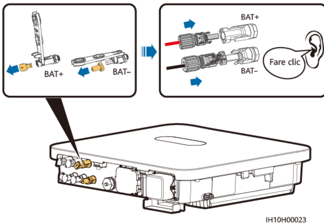
Figura 5-12 Collegamento dei cavi della batteria
