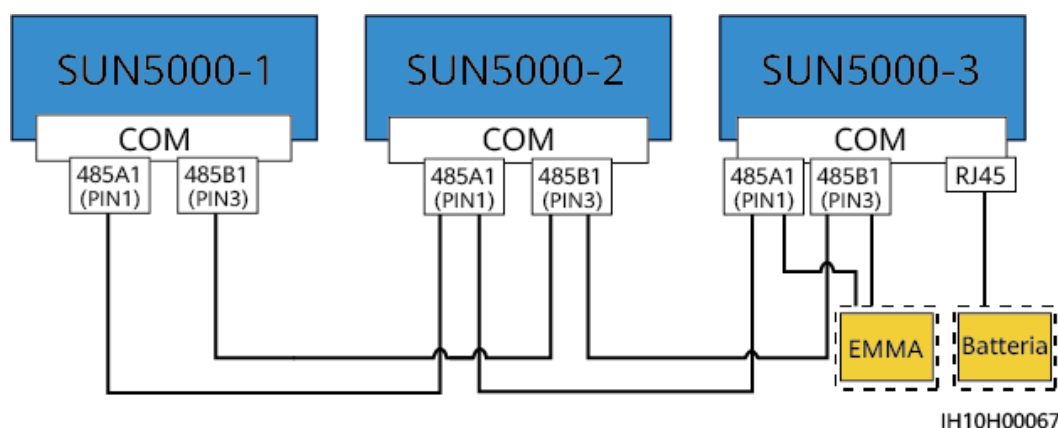
Figura 5-16 Collegamento in rete di EMMA (i riquadri tratteggiati indicano i componenti opzionali)
