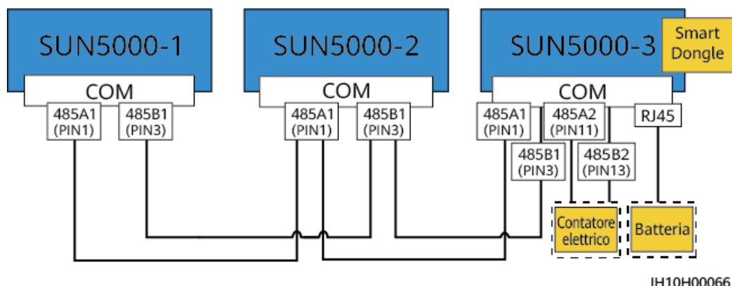
Figura 5-15 Collegamento in rete dello Smart Dongle (i riquadri tratteggiati indicano i componenti opzionali)
